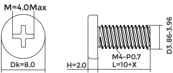
壁掛螺絲規格：M4*(10+X)mm (X=壁掛式支架的厚度)
