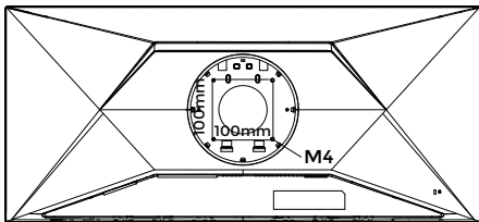
Specificatie van schroeven voor muurbevestiging: M4*(10+X) mm (X=dikte van haak voor muurbevestiging)
